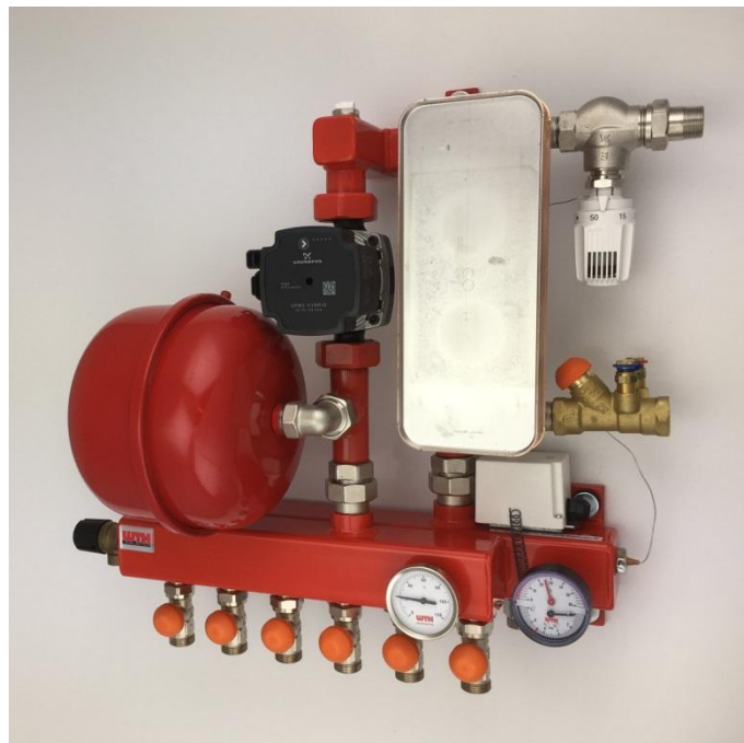
Afbeelding: LTSW-N 6 groeps voorzien van WW-module
